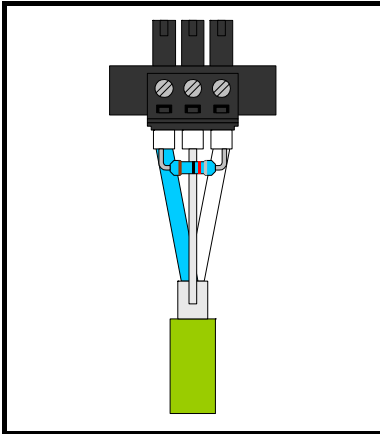
Рис. 3-4 Согласование сети CTNet
