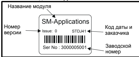
Рис. 2-2 Шильдик SM-Applications
