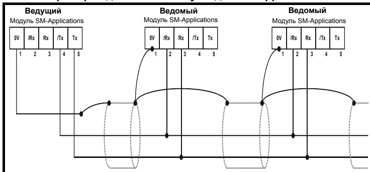
Рис. 9-1 Пример подключения CTSync для SM-Applications
