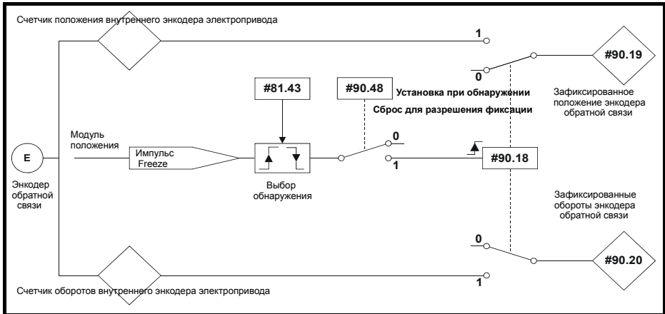
Рис. 8-4 Вход фиксации энкодера обратной связи в Apps Lite/Apps Lite V2 и Digitax St Indexer
