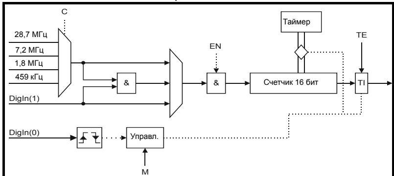
Рис. 5-1 Логическая схема таймера
