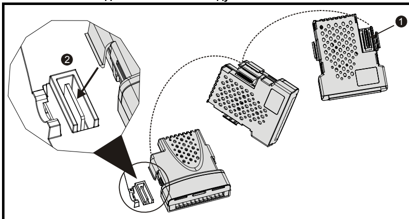
Рис. 3-1 Установка дополнительного модуля
