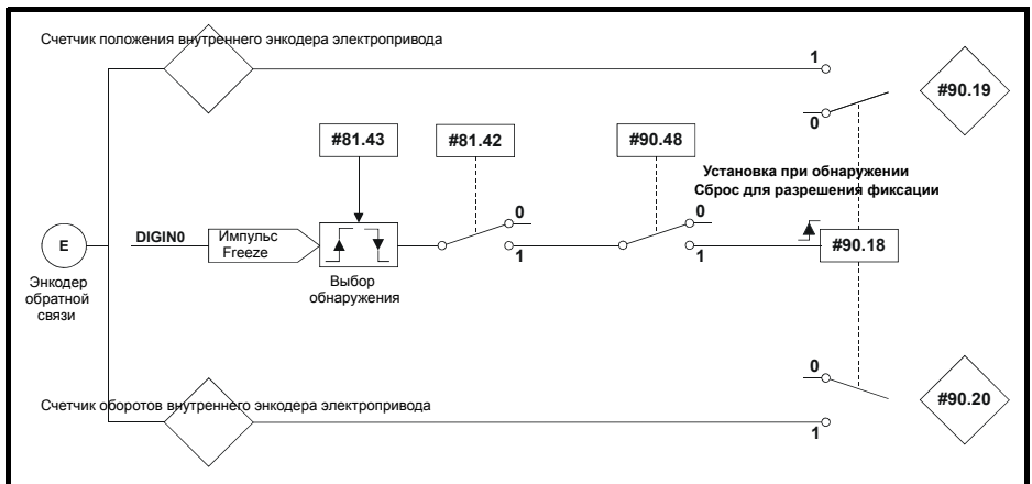
Рис. 8-2 Фиксация энкодера обратной связи в SM-Apps/SM-Apps Plus/Digitax ST Plus
