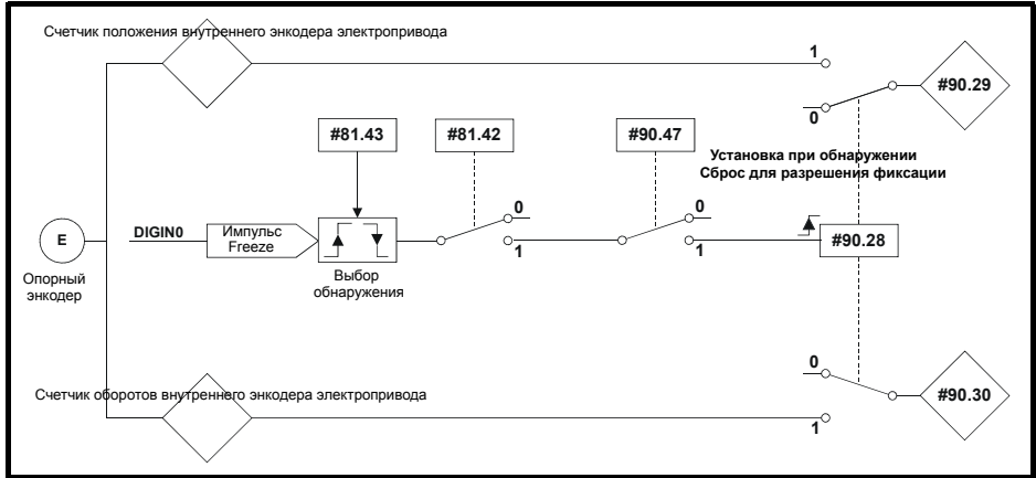
Рис. 8-1 Фиксация опорного энкодера в SM-Apps/SM-Apps Plus/Digitax ST Plus
