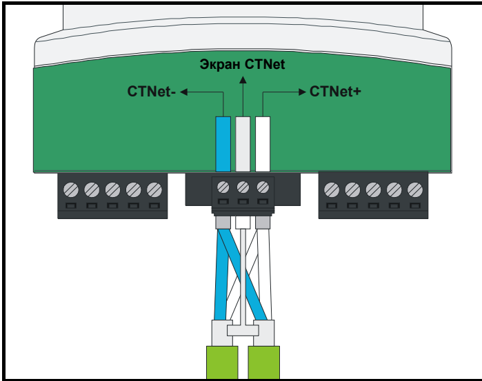
Рис. 3-3 Подключение сети CTNet
