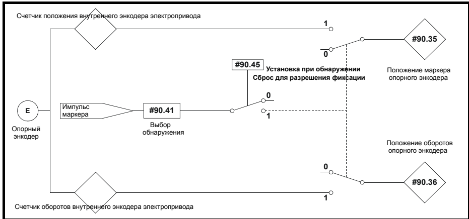
Рис. 8-5 Опорный маркер второго процессора
