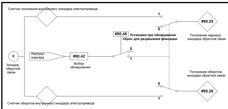
Рис. 8-6 Маркер обратной связи второго процессора
